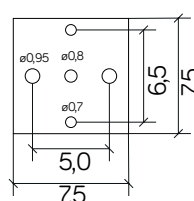
podstawa / base
