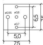
podstawa / base
