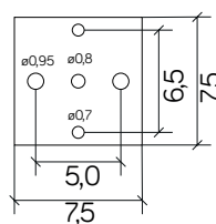
podstawa / base
