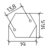
podstawa / base
